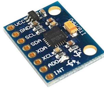
(d) Motion sensor board
